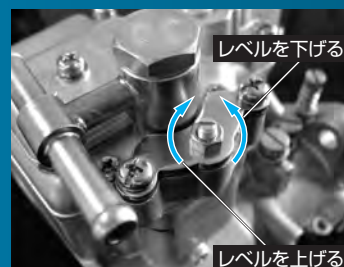
●フロートレベルの調整 エンジンの好不調は、フロートレベルで左右されます。このスクリューを廻すだけで容易に調整できます。
